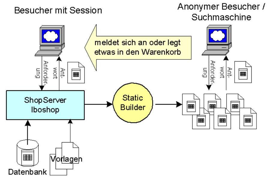
Abbildung: Zusammenspiel zwischen den dynamischen und statischen ShopPilot Seiten
